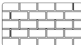
Behúňova väzba
